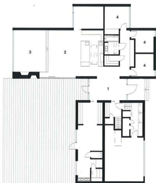
ENTRÉPLAN 1:300
